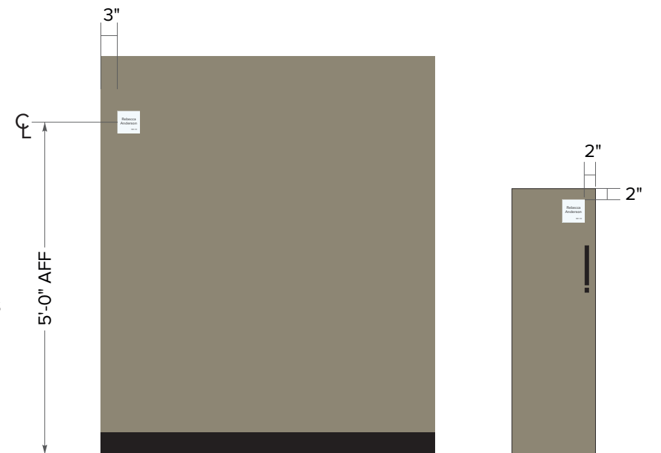
CUBICLE INSTALL (TYP.) SCALE: 1/2" = 1'-0"
