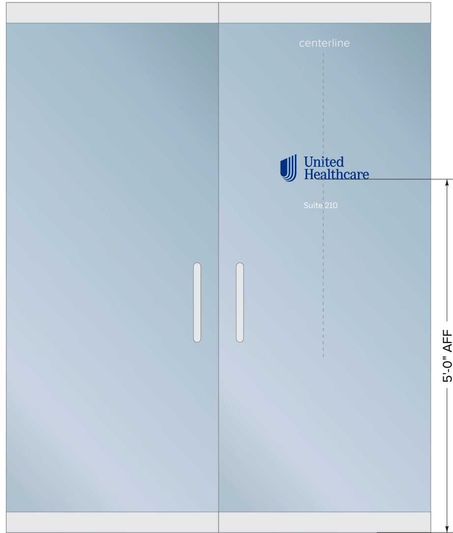
scale: 3/4" = 1'-0"
